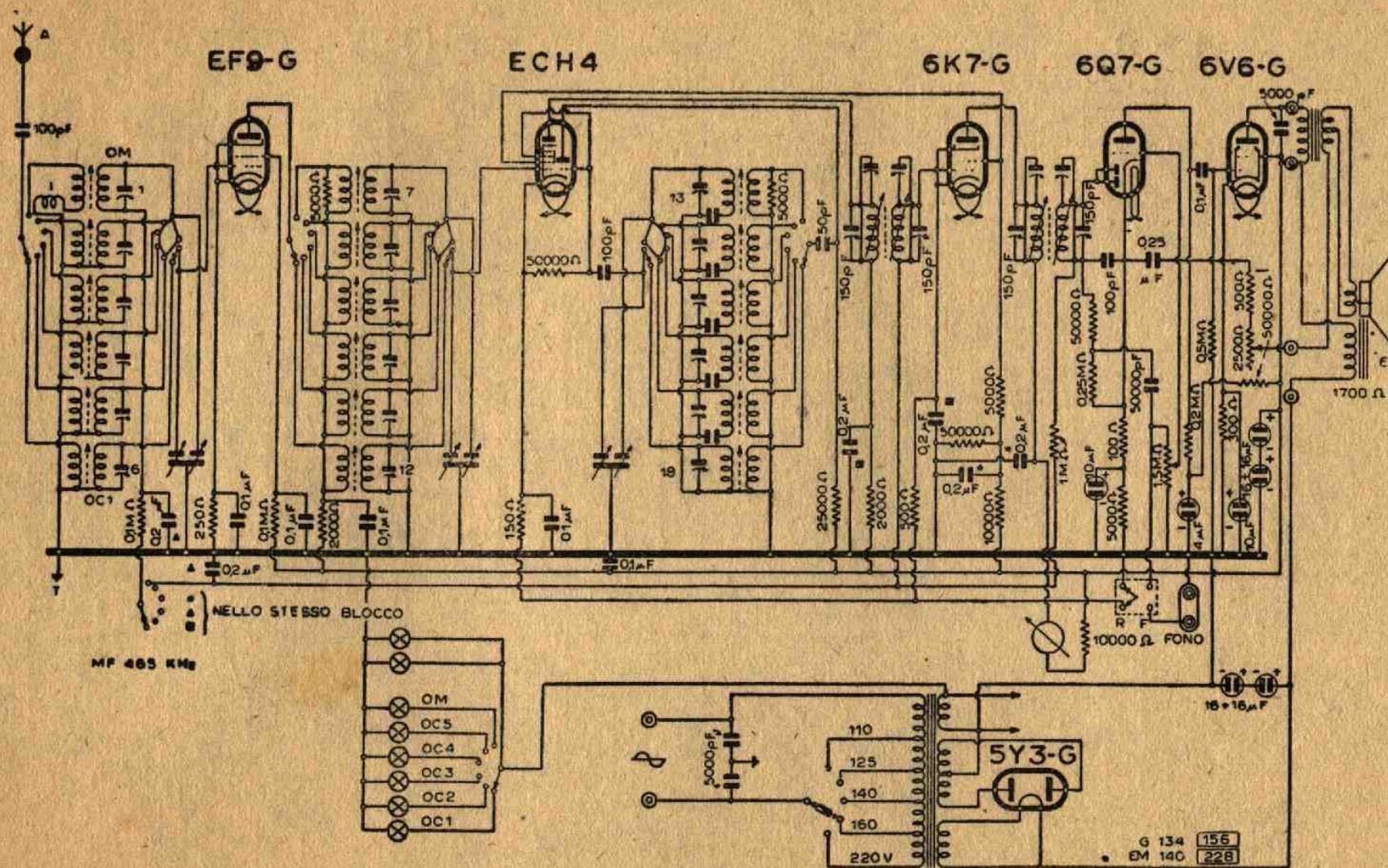
Lo schema elettrico del mod. 615
